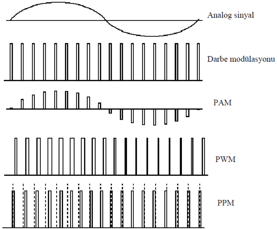
Şekil 2.2 Darbe modülasyonu çeşitleri
