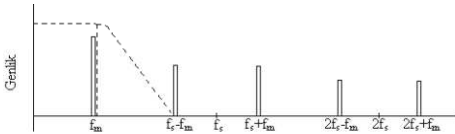
Şekil 2.5: Örneklenmiş sinyalin frekans spektrumu
