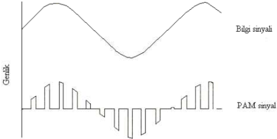
Şekil 2.6 Tabii örneklenmiş PAM sinyal
