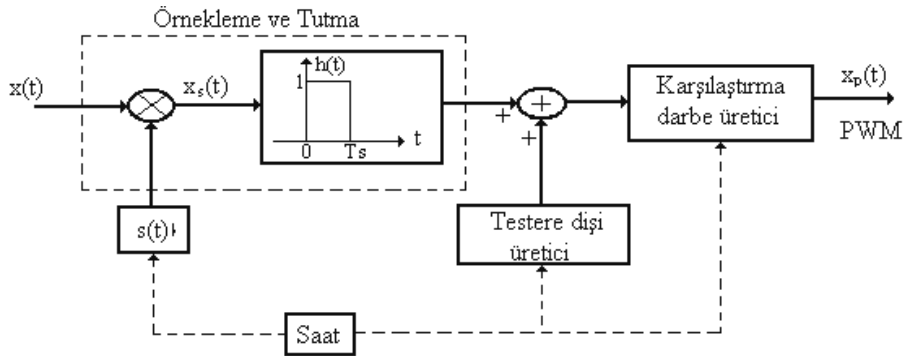
Şekil 2.12: PWM dalgasının üretiminin blok diyagramı
