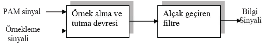
Şekil 2.10: PAM demodülatörü blok diyagramı
