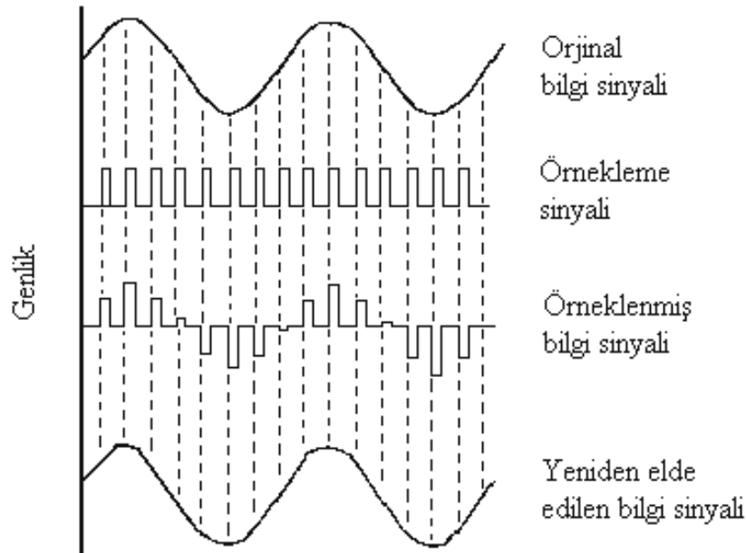
Şekil 2.3: Yeterli sayıda örneklenmiş sinyal
