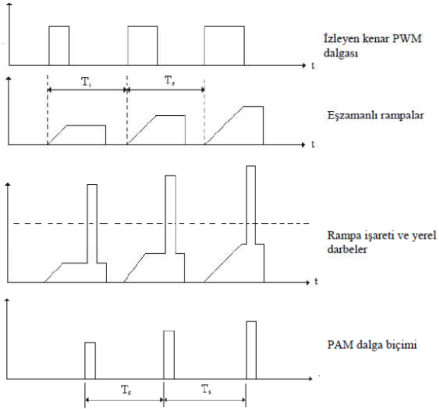
Şekil 2.14: PWM dalgasının PAM dalgasına dönüştürülmesi
