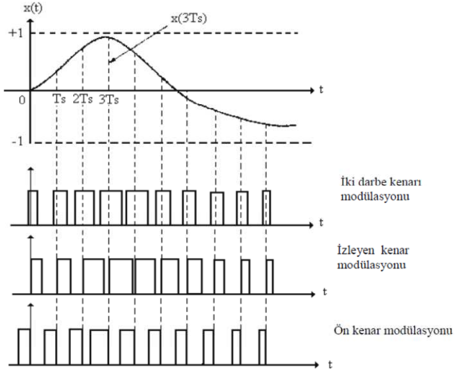
Şekil 2.11: PWM modülasyonu dalga biçimleri
