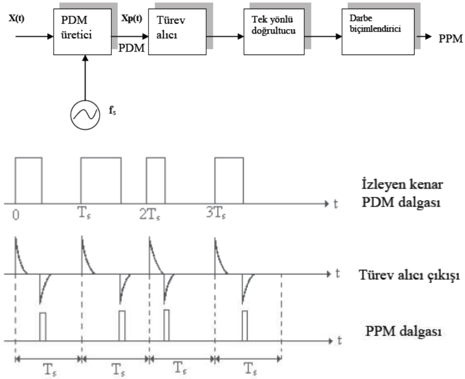
Şekil 2.15: PPM dalgasının üretim aşamaları
