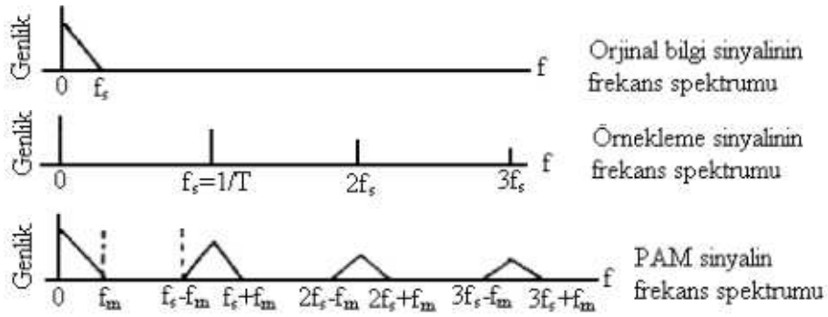
Şekil 2.8: PAM sinyal frekans spektrumu
