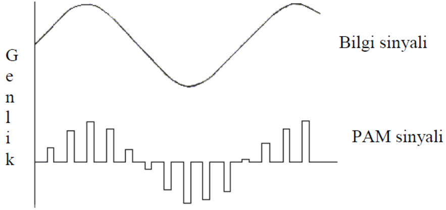
Şekil 2.7: Düz tepe örneklenmiş PAM sinyal
