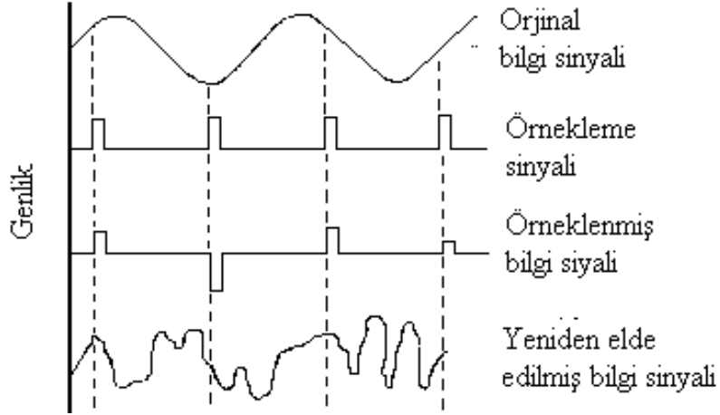
Şekil 2.4: Yetersiz sayıda örneklenmiş sinyal
