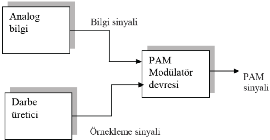
Şekil 2.9: PAM modülatörü blok diyagramı
