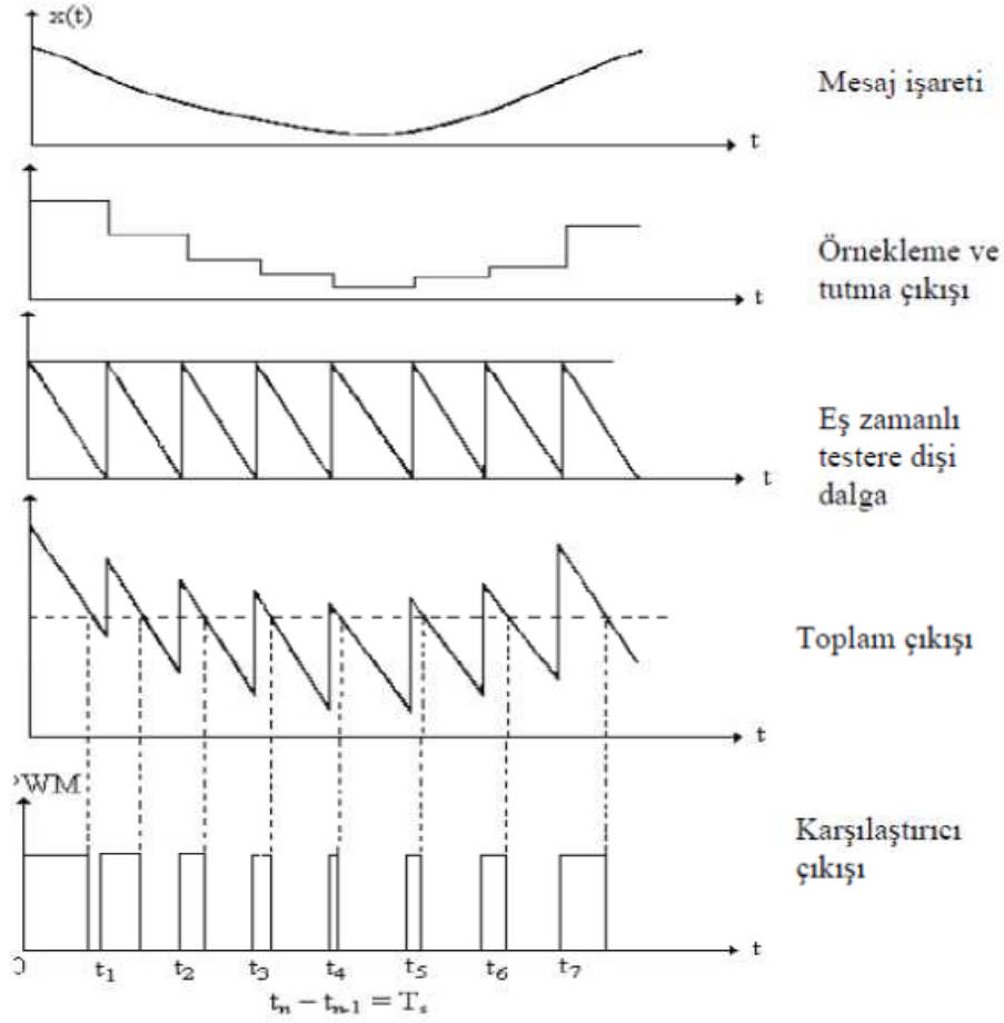
Şekil 2.13: PWM işaretinin üretilmesi
